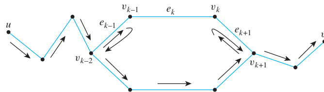
Figura 10.5.4 Un ejemplo de un camino de u a w que no incluye a la arista e_k
